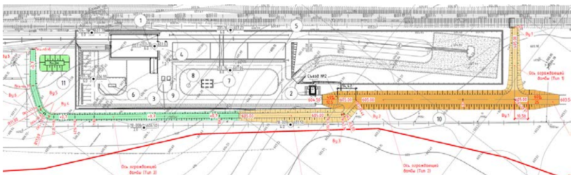
Рисунок 2. План ограждающей дамбы
