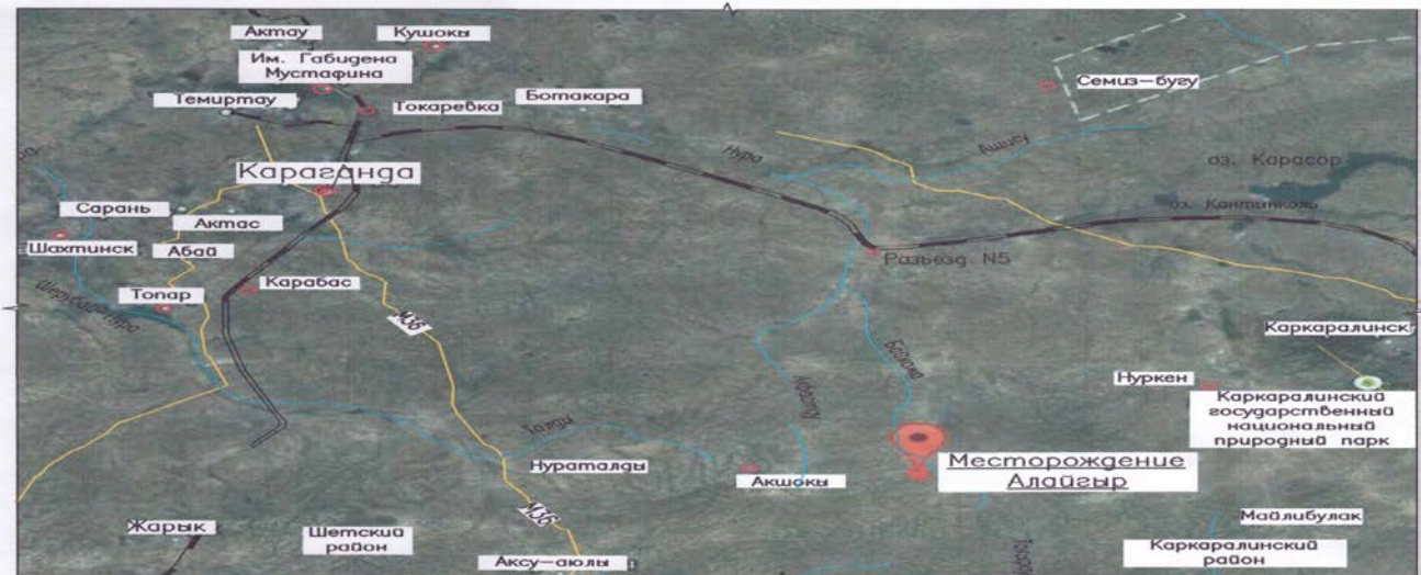
Рисунок 1. Месторасположение месторождения Алайгыр.
